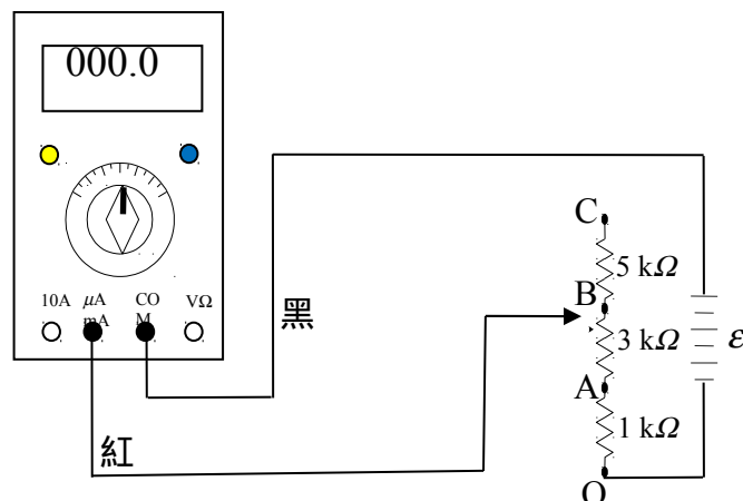
圖三：直流電流測定示意圖
