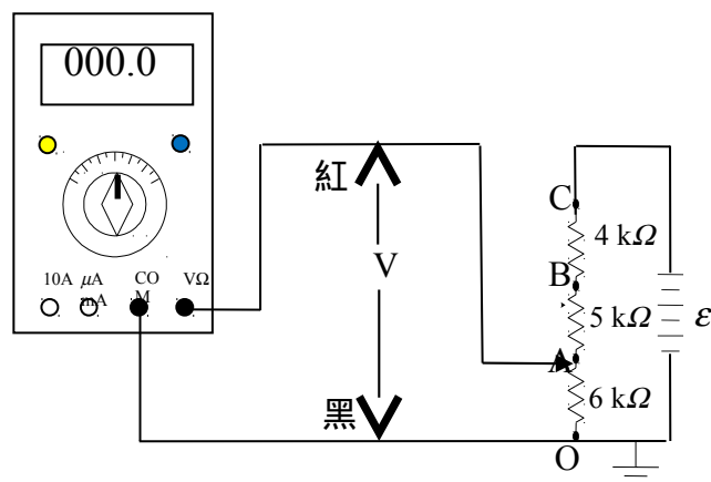
圖二：直流電壓測定示意圖
